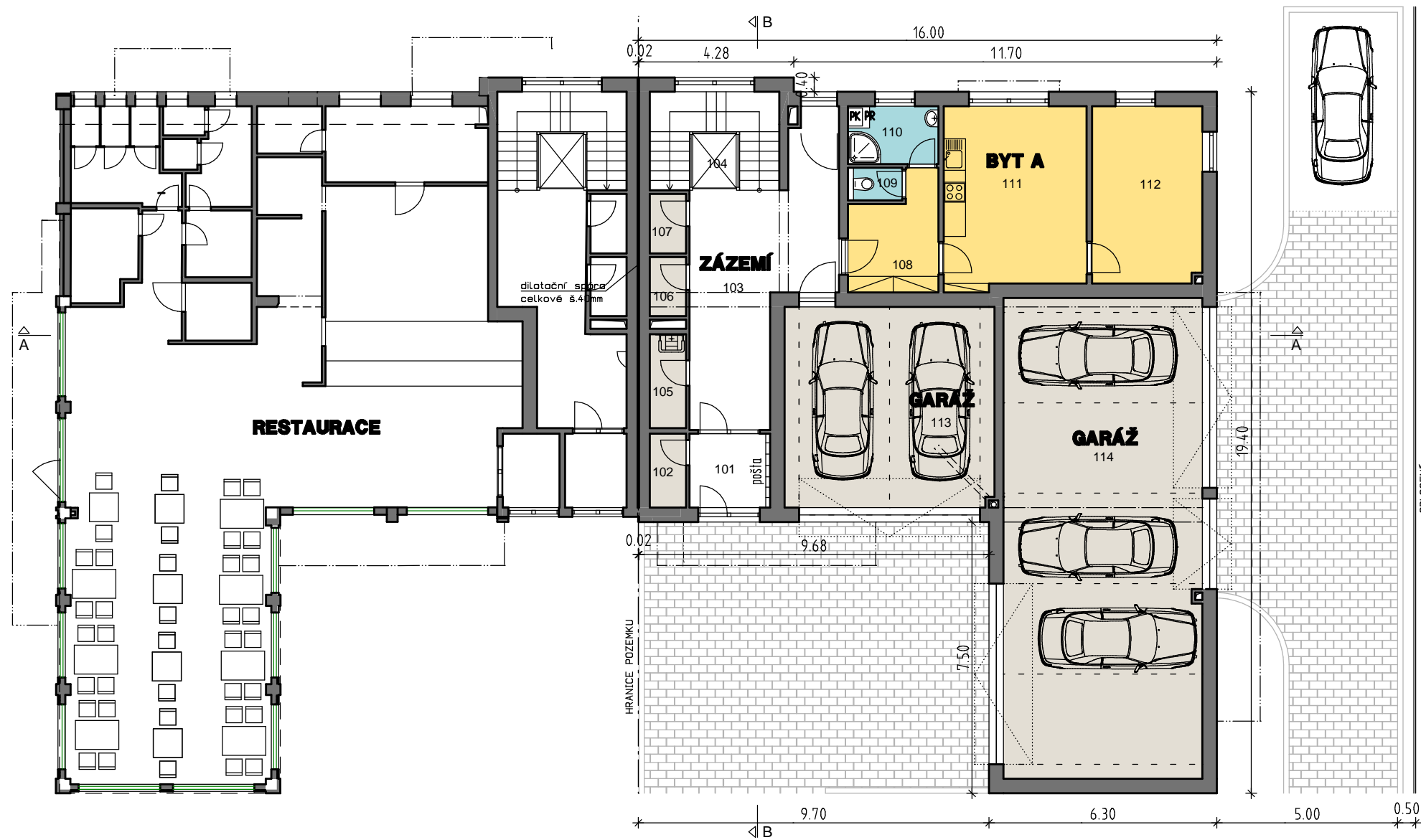
LEGENDA MÍSTNOSTÍ - 1.NP
